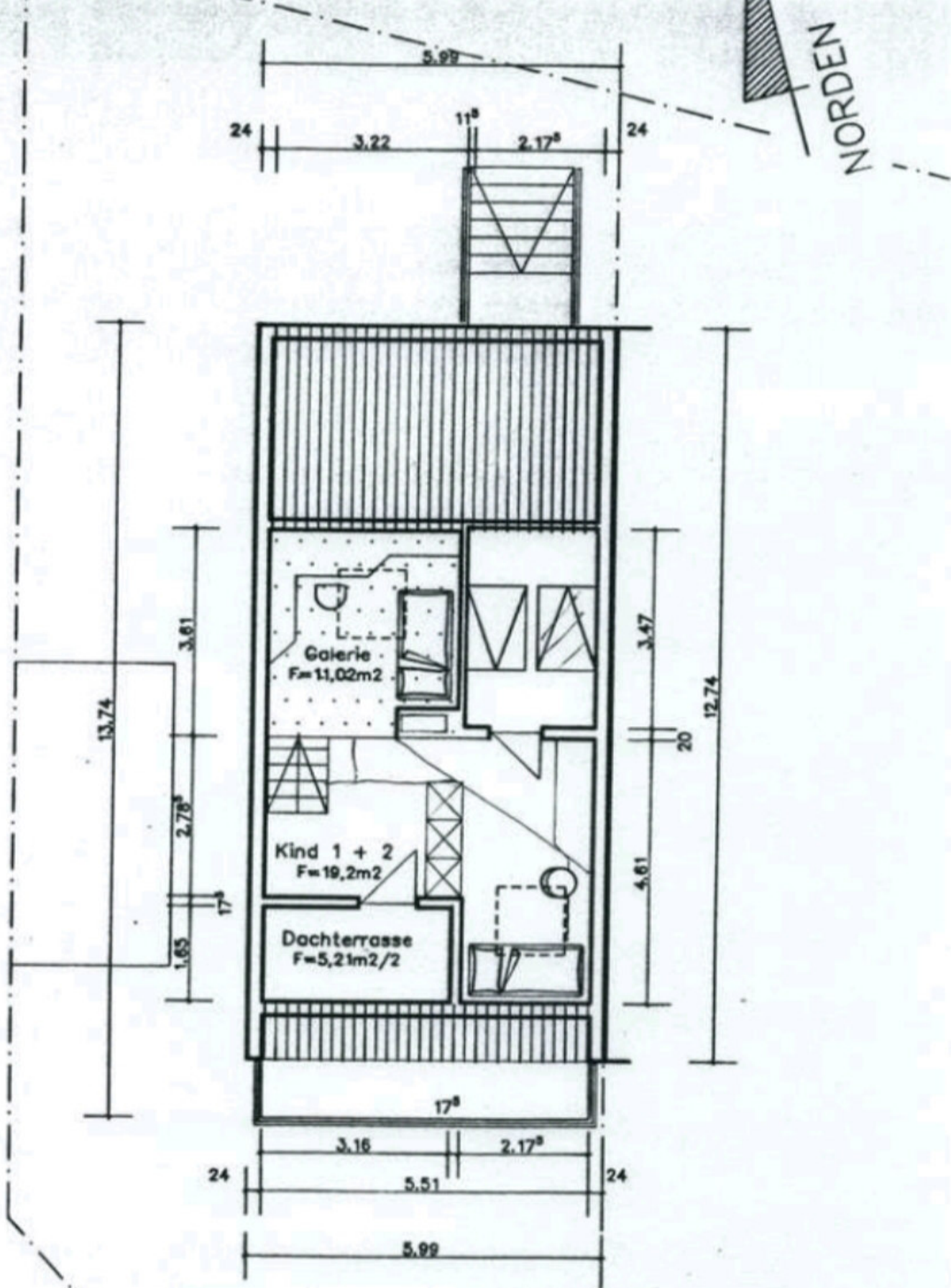
Grundriss Dachgeschoss M 1 : 100 (gepunktete Fläche liegt ein halbes Geschoss höher)
