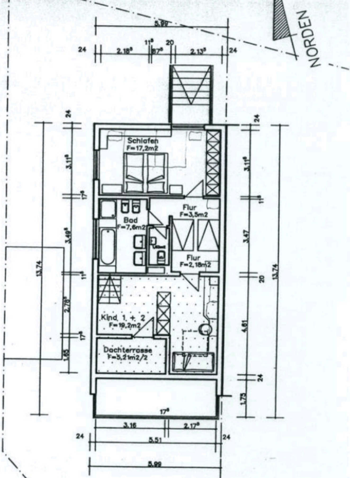
Grundriss Obergeschoss M 1 : 100 (gepunktete Fläche liegt ein halbes Geschoss höher)
