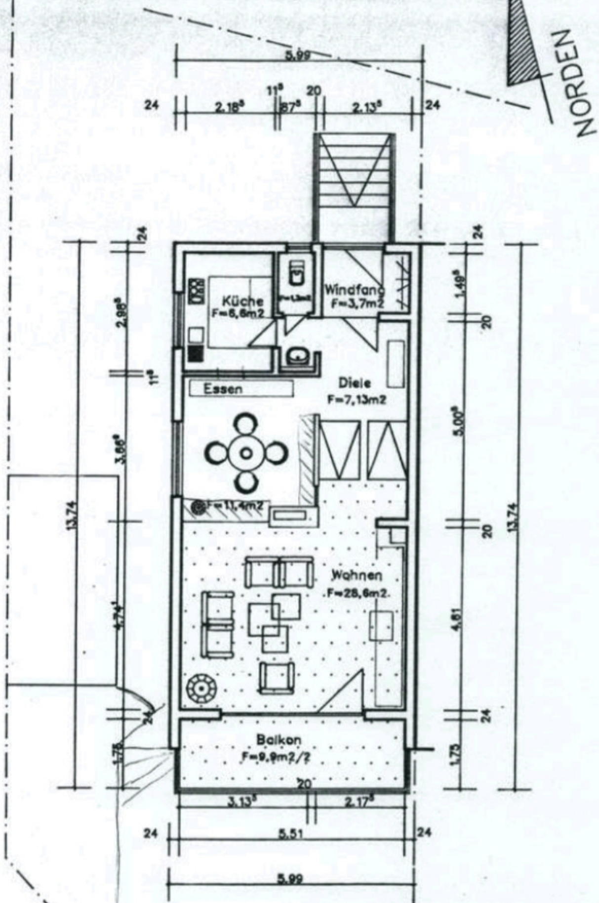
Grundriss Erdgeschoss M 1 : 100 (gepunktete Fläche liegt ein halbes Geschoss höher)
