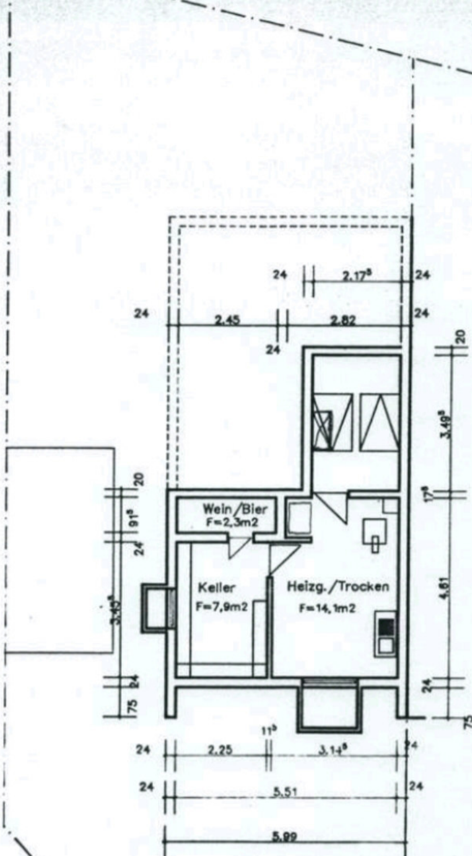
Grundriss Untergeschoss M 1 : 100
